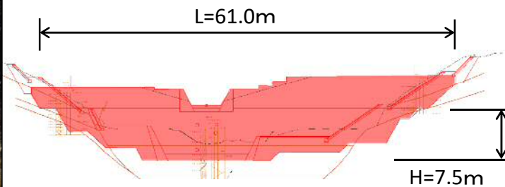
堰堤一般図
