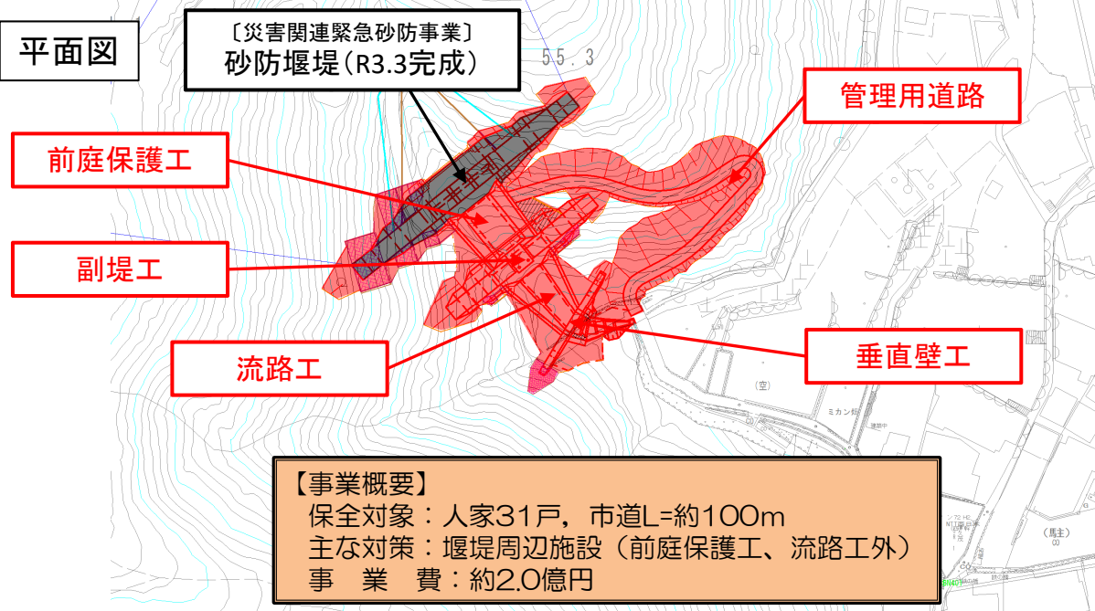
堰堤一般図
