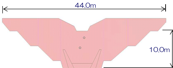
堰堤一般図
