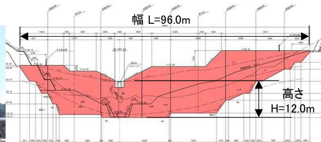
堰堤一般図
