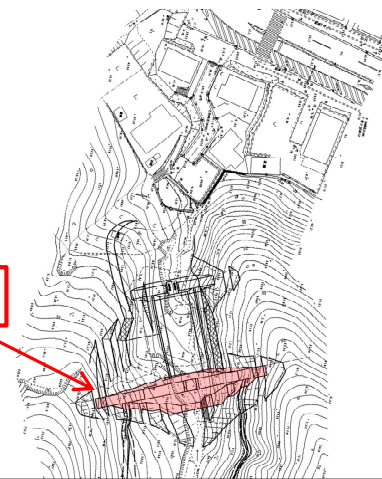
砂防堰堤
