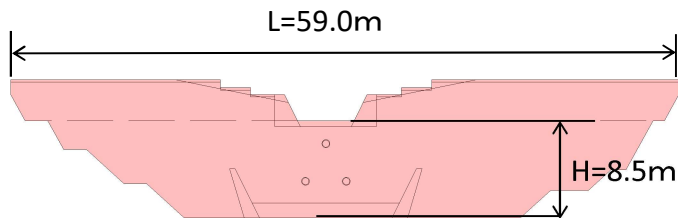
堰堤一般図
