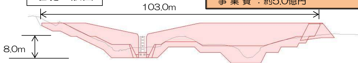
堰堤一般図
