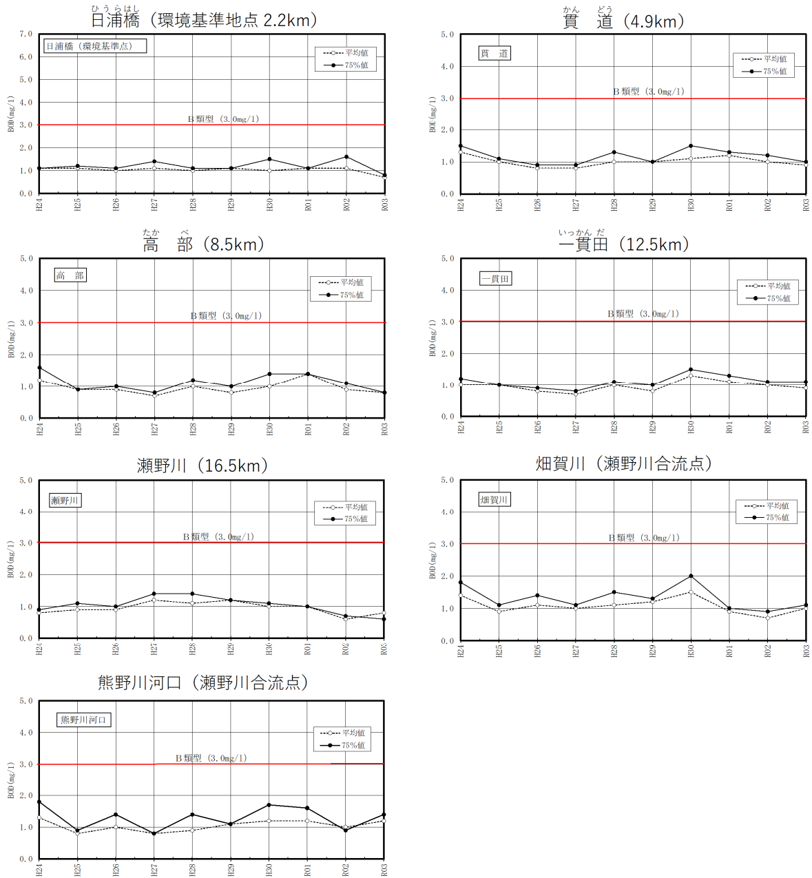
図-1.2.3 瀬野川におけるBOD（平均値・75%値）の推移
