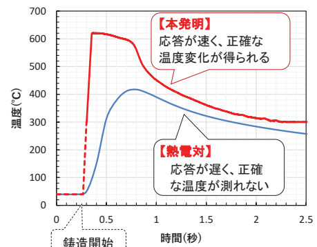
【ダイカストにおける测温結果】
