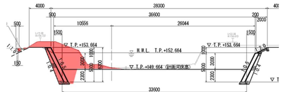
標準断面図 (A-A)
