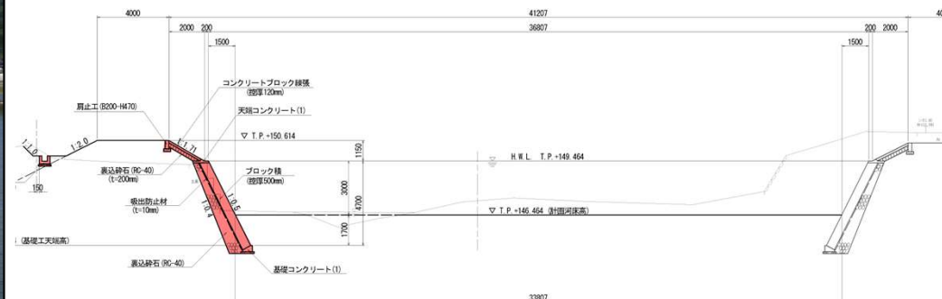
標準断面図 (A-A)
