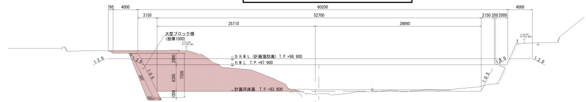
標準断面図 (A-A)
