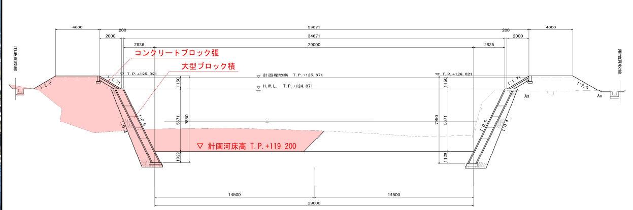
標準断面図 (A-A)
