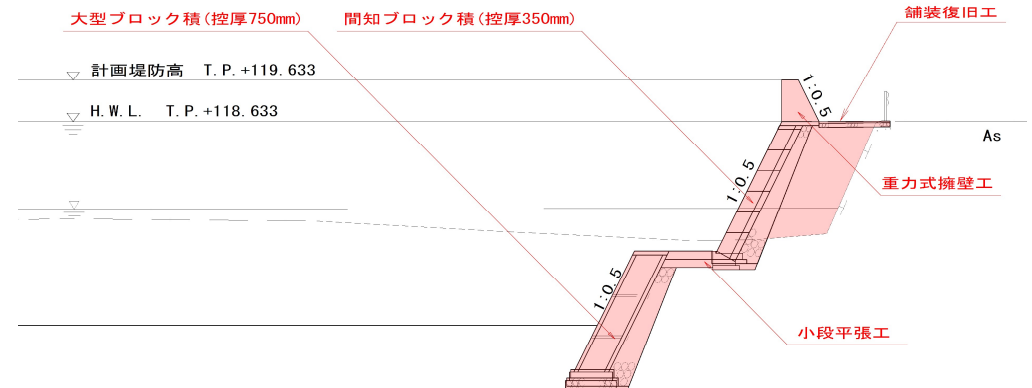
標準断面図 (A-A)
