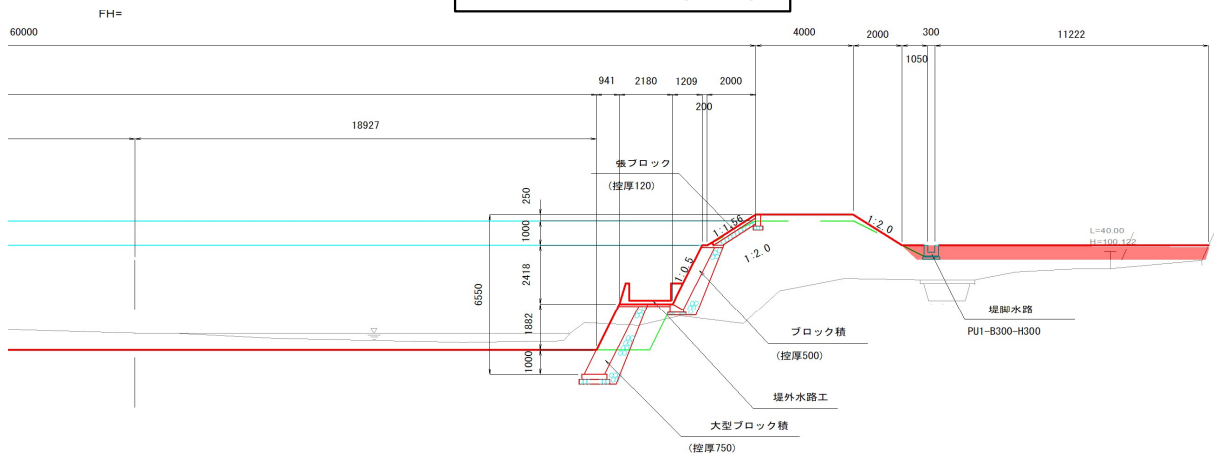
標準断面図 (D-D)
