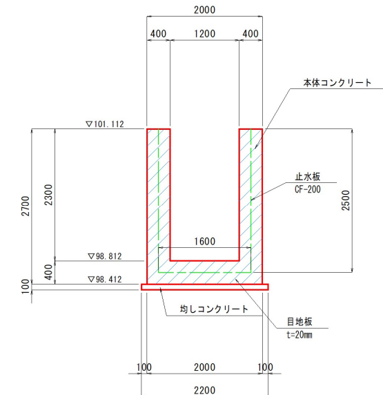
現場打水路構造図
