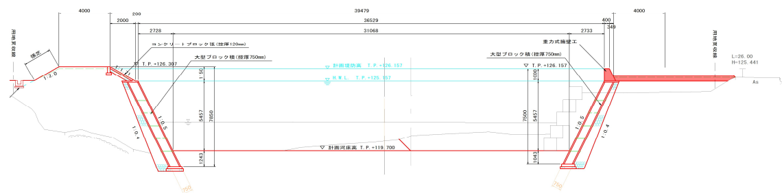
標準断面図 (C-C)
