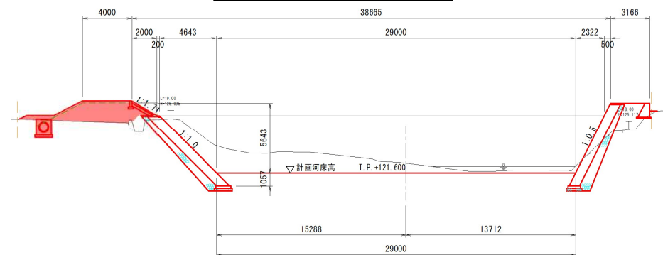
標準断面図 (B-B)
