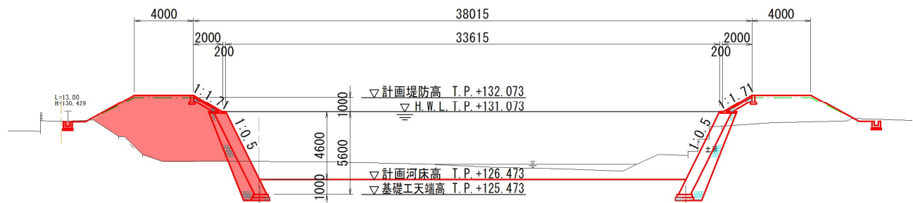
標準断面図 (A-A)
