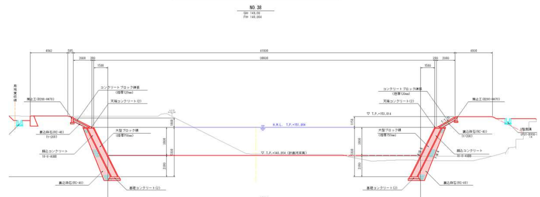
標準断面図 (A-A)
