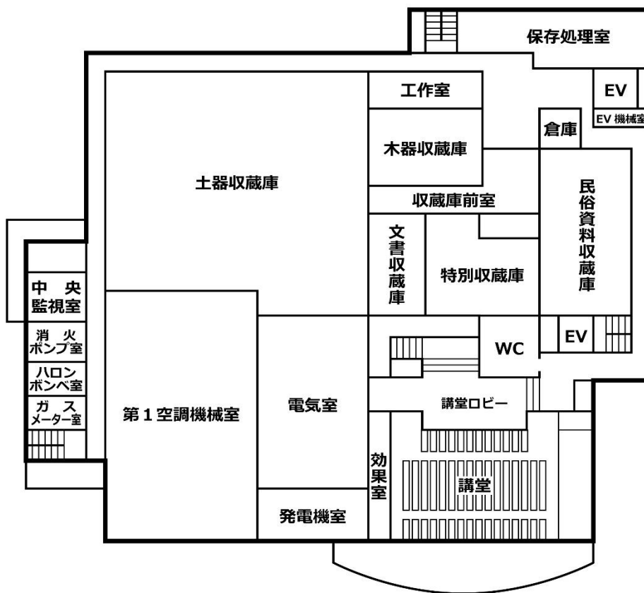
地階平面図
