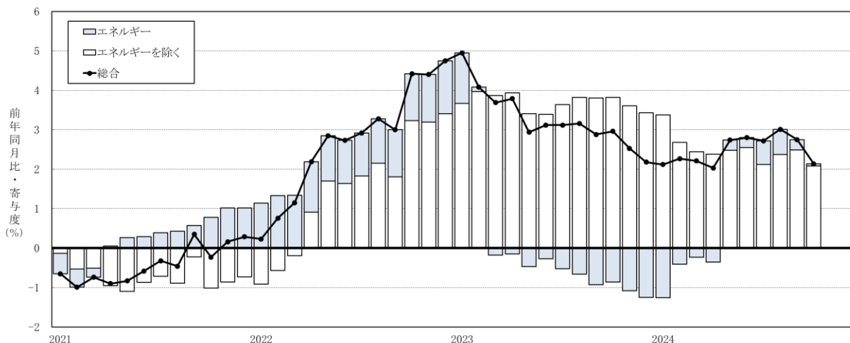
図6 総合指数の前年同月比に対するエネルギー寄与度の推移 2021.1～2024.10
