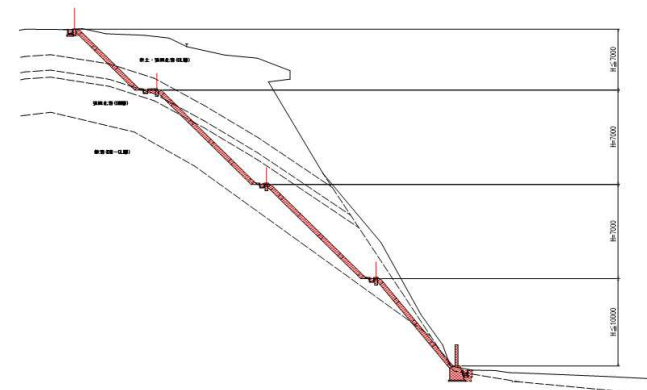
標準断面図
