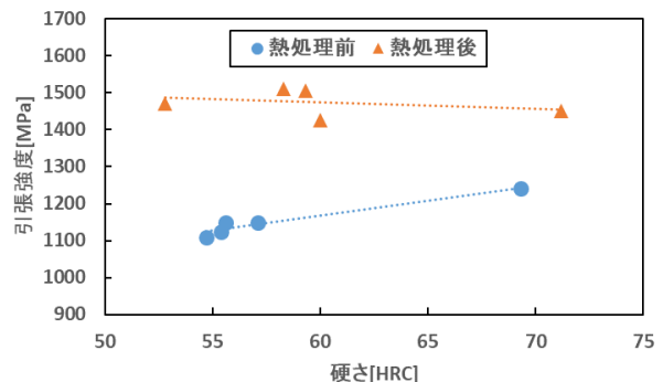
引張強度
