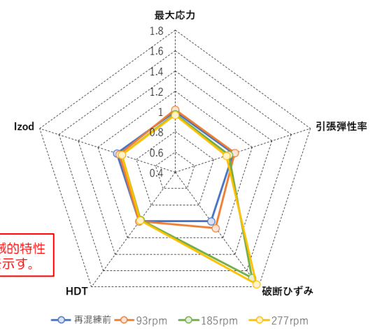
リサイクルペレットでのスクリュ回転数と各種物性の関係※
