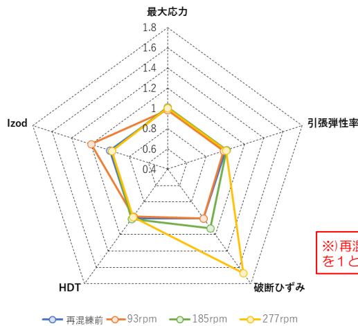
バージンペレットでのスクリュ回転数と各種物性の関係※
