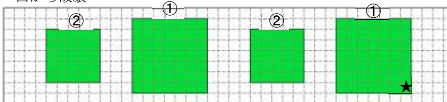
図Ⅳ. 2. 1-4(2) 断層モデル:中央構造線断層帯(讃岐山脈南縁西部区間)
