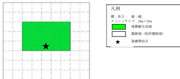
図IV. 2. 1-5 断層モデル：どこでも起こりうる直下の地震
