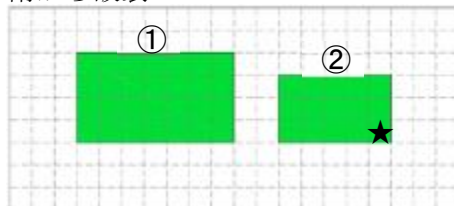
図IV. 2. 1-4(10) 断層モデル：広島湾－岩国沖断層帯
