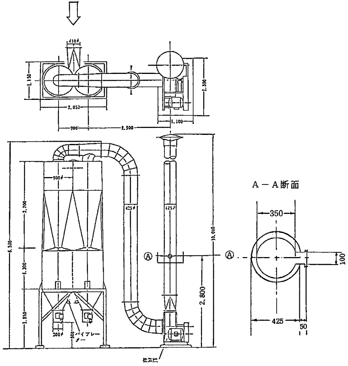
(サイクロン集じん装置)
