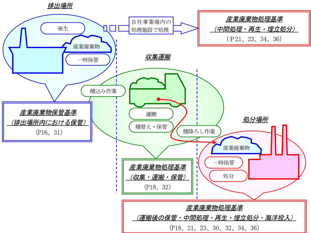
図表 13 廃棄物の発生から適正処理までの過程と適用基準
