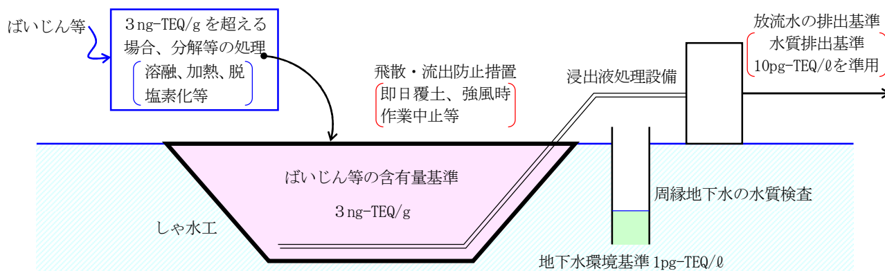
図表 43 最終処分場における措置
