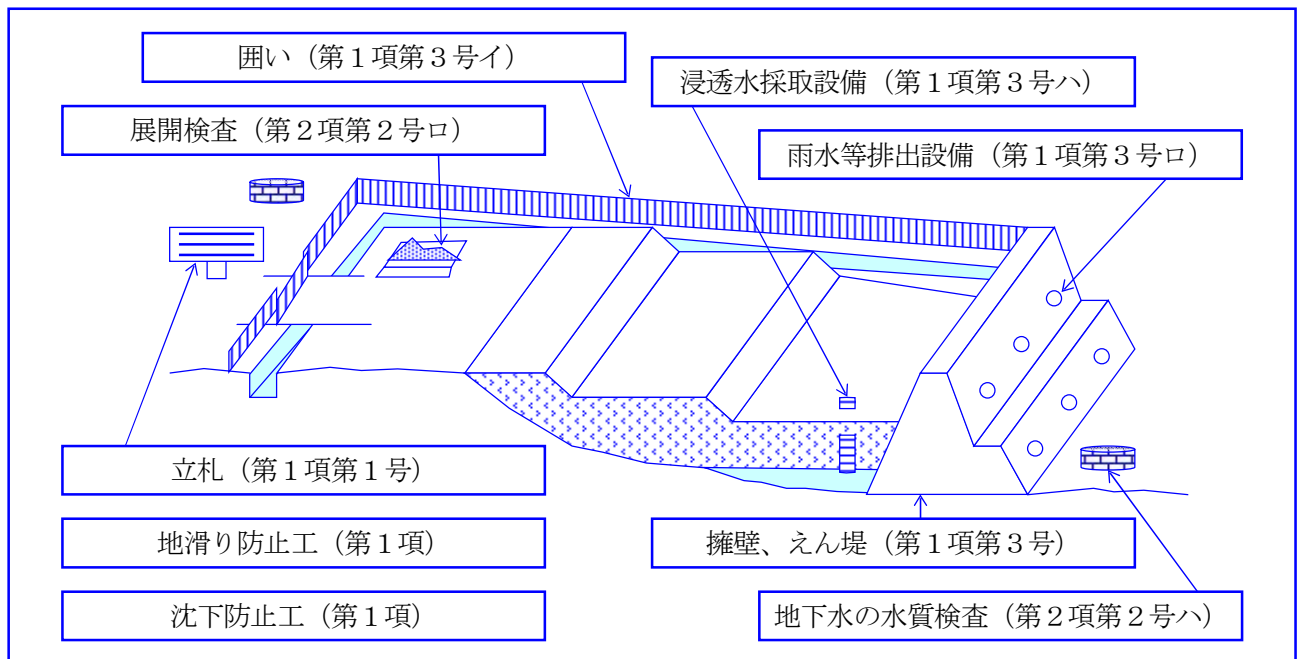
図表 27 管理型最終処分場の構造等（最終処分基準省令第 2 条）
