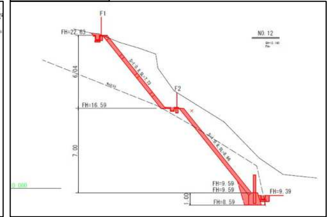
標準断面図
