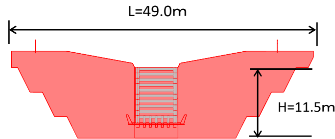
堰堤一般図
