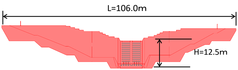
堰堤一般図
