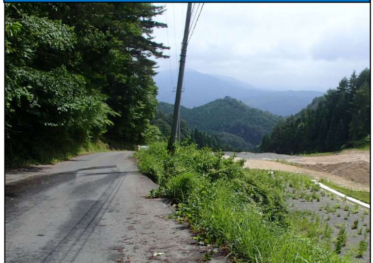
【施工前】
