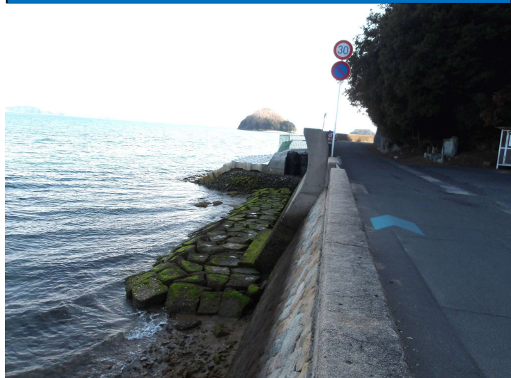
【施工状況】
