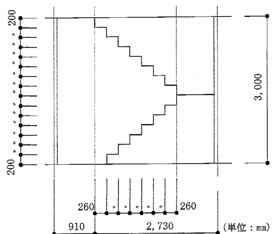
図2 断面計画図
