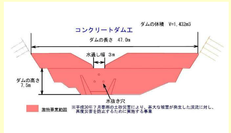
【正面図】
