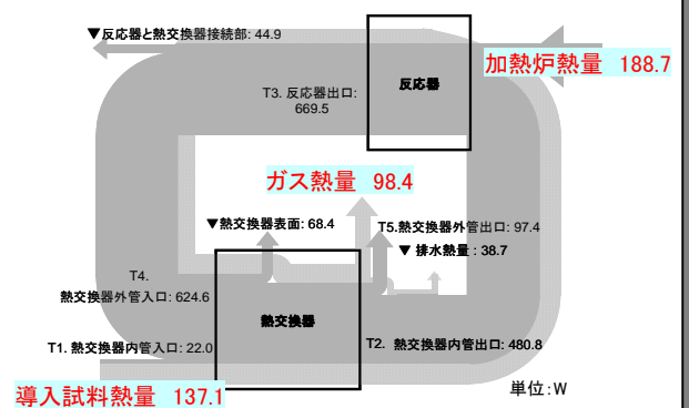
8 wt%間欠運転のエネルギー収支 (実験値、▼熱損失)
