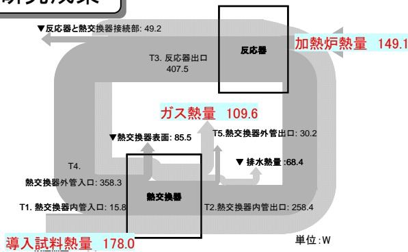
8 wt%非間欠運転のエネルギー収支 (2 wt%の結果から算出、▼熱損失)
