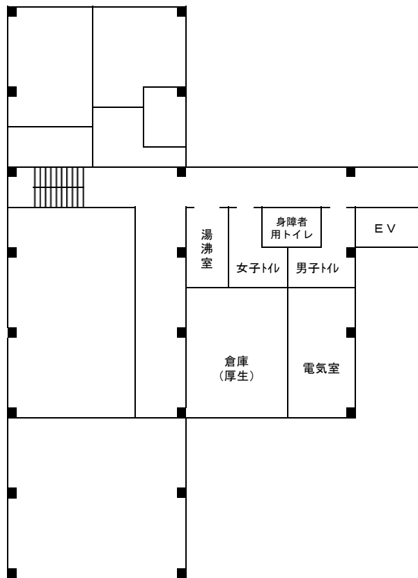
2階平面図
