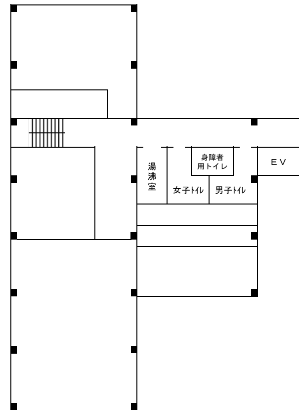
3階平面図
