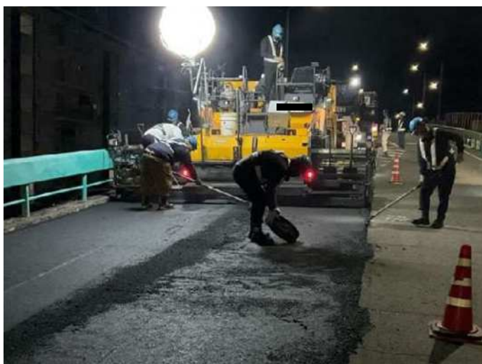
一般国道１８６号 舗装補修（大竹市北栄）
