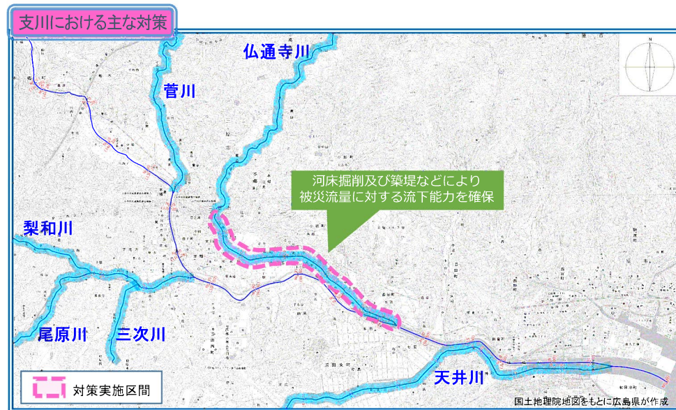
整備位置図
