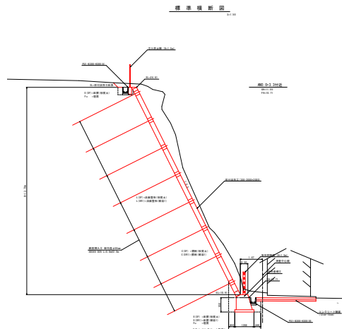
標準断面図
