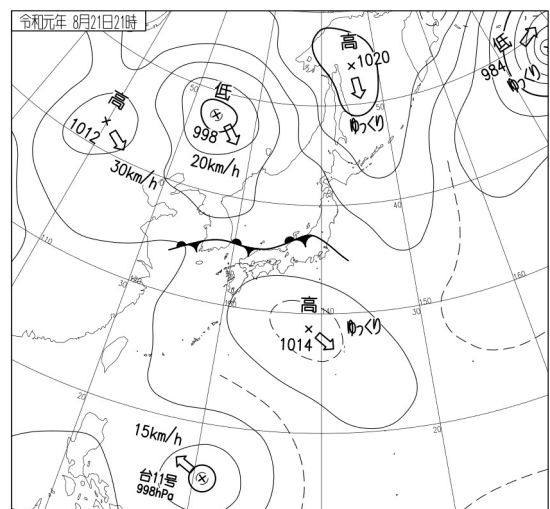
地上天気図
