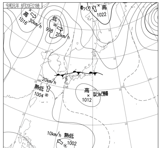
地上天気図
