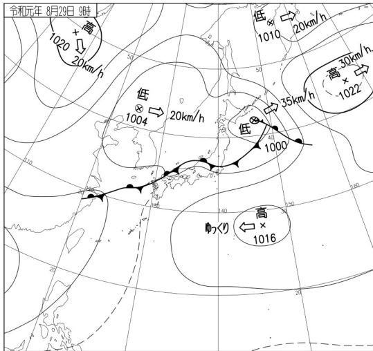
地上天気図
