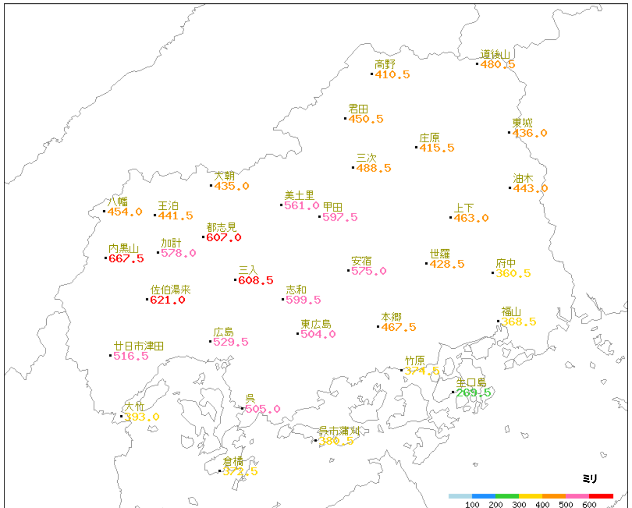
アメダス地点の降水量分布図（12日間合計）
