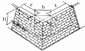
(a) 立体図
